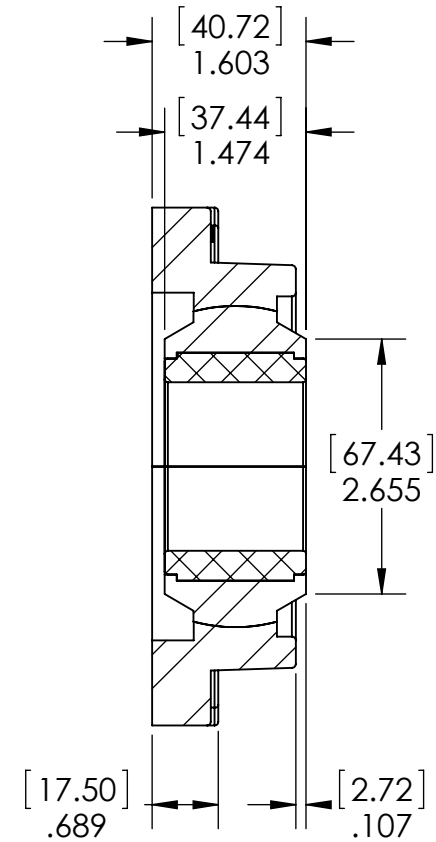
SECTION T-T SCALE 1 : 2
